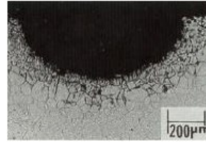
Alloy 800H
